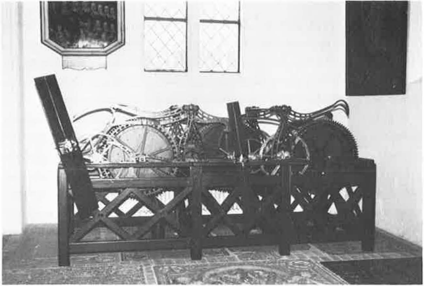
Tårnmur i Nyborg Kirke 1847-1954, udført af den københavnske tårnmurer H. Larsen Kyhl. Værket står nu i kirkens nordre tværskib.
